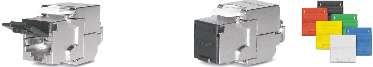
RJ45 module KS-T Plus 1/8 tool-less Cat.6A (IEC), afgeschermd, met stofluikje
