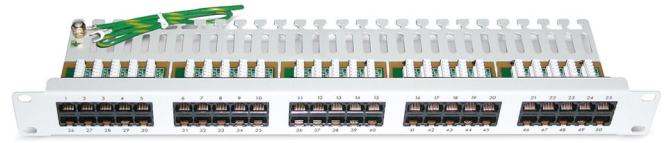
Telefoniepaneel CU 50/4
