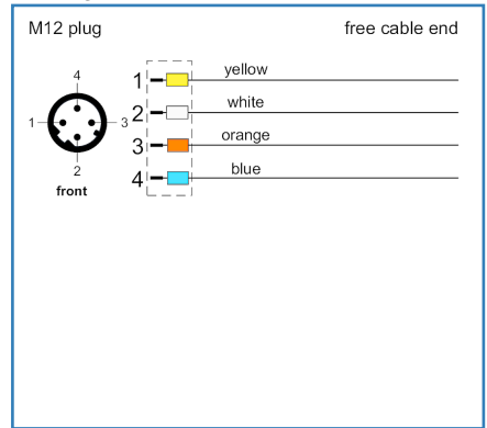
Wiring
