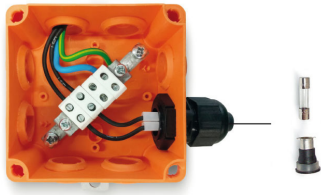
Zekeringselement aanbouw M25/2A
